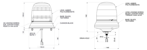
3 Bolt
